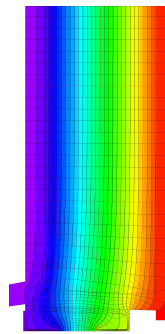
Isothermengrafik
